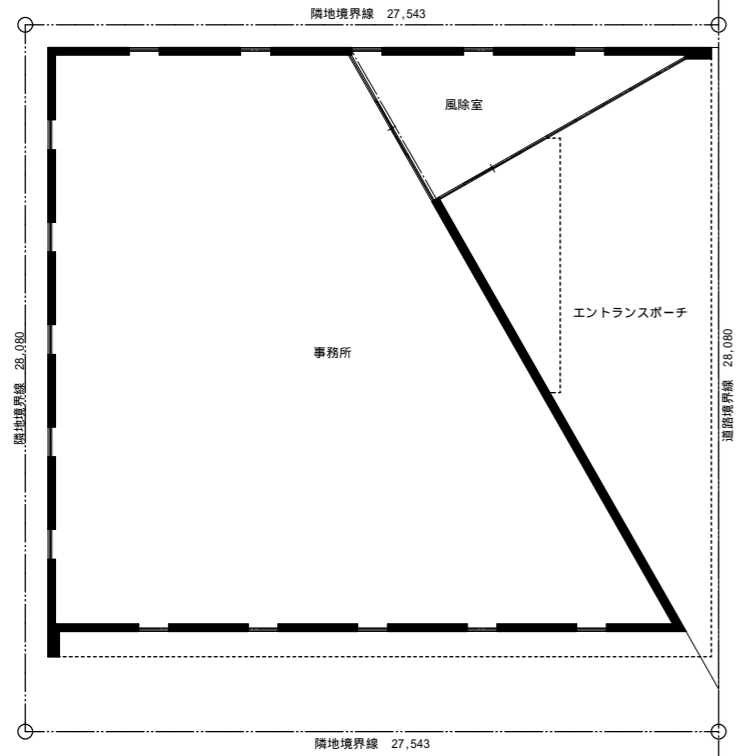
1 階平面図
