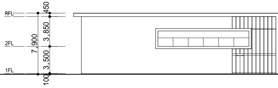
南側 立面図
